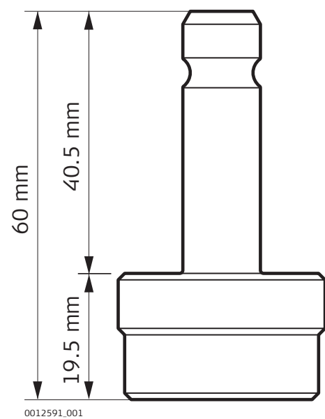
Адаптер GAD50
